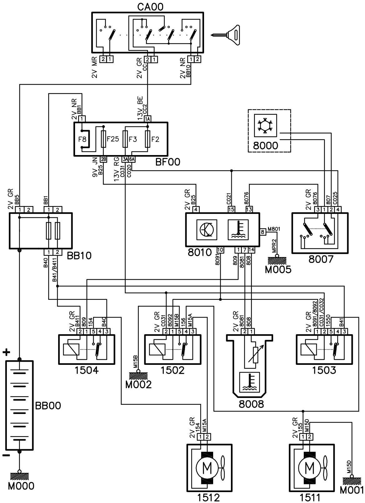
دیاگرام شماتیک مدار خنک کننده موتور با کنترل یونیت فن
